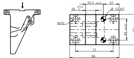
008 (8090) CUNEO / WEDGE / DRUCKSTÜK
