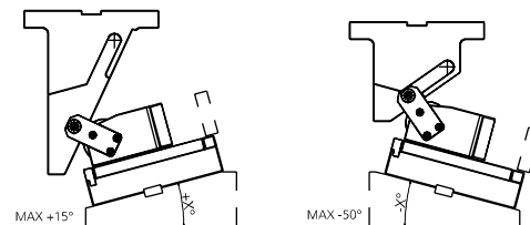
008 (8090) CUNEO / WEDGE / DRUCKSTÜK
