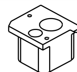
8021.0002... PORTA PUNZONE / PUNCH HOLDER / TRÄGERPLATTE
