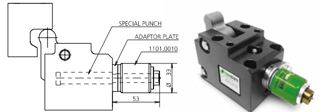
8124.0140.0210 KIT ADATTAMENTO STARK STRIPPER / STARK-STRIP ADAPTION KIT / STARK-STRIP ADAPTIONSSATZ
